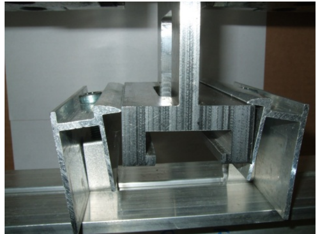
Bild 8 Versagen von Randklemmen durch Abrutschen
