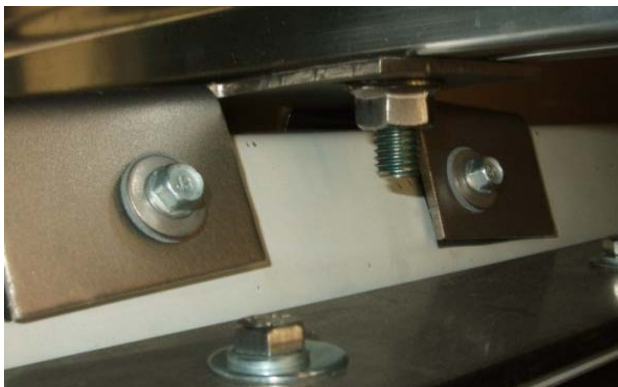
Bild 14 Trapezzschellen mit seitlicher Fixierung am Steg
